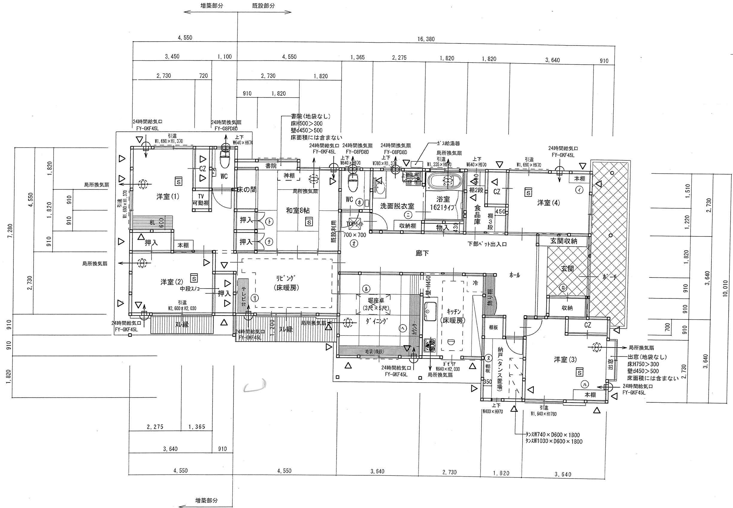
増改築後平面図 S=1/100
